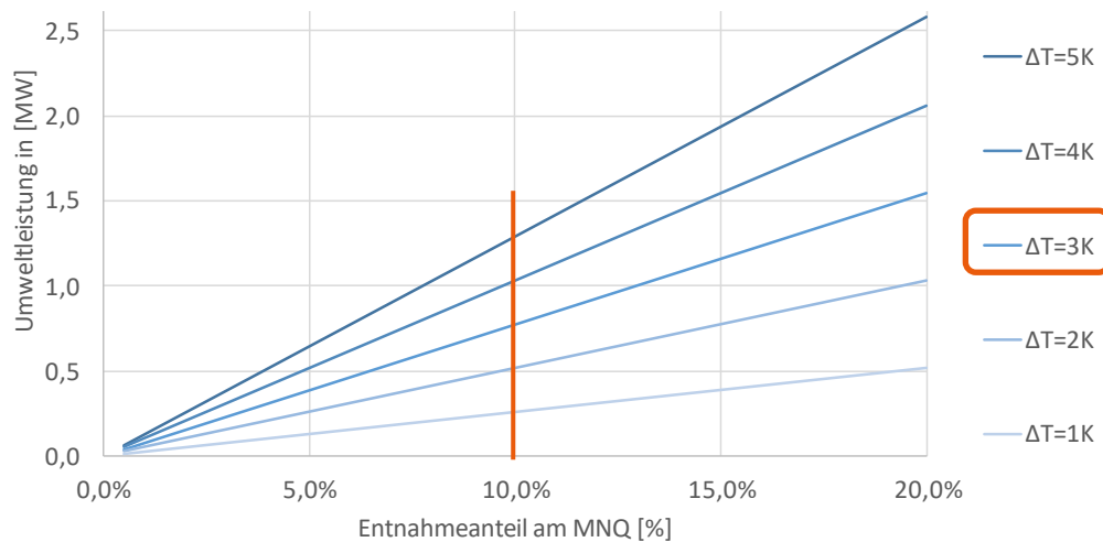
Abbildung 32: Umweltleistung am Wärmetauscher in der Unteren Steinach in Abhängigkeit der Entnahmemenge und Temperaturspreizung
