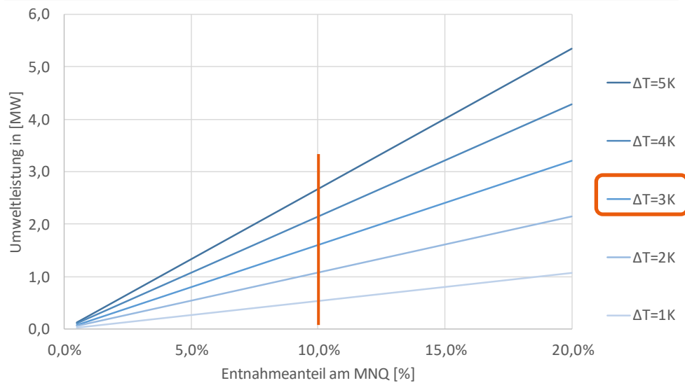
Abbildung 33: Umweltleistung am Wärmetauscher in der Schorgast in Abhängigkeit der Entnahmemenge und Temperaturspreizung
