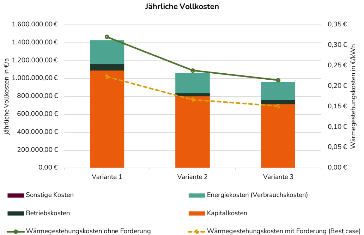
Abbildung 52: Variantenvergleich JGK und WGK Untersteinach Zentrum
