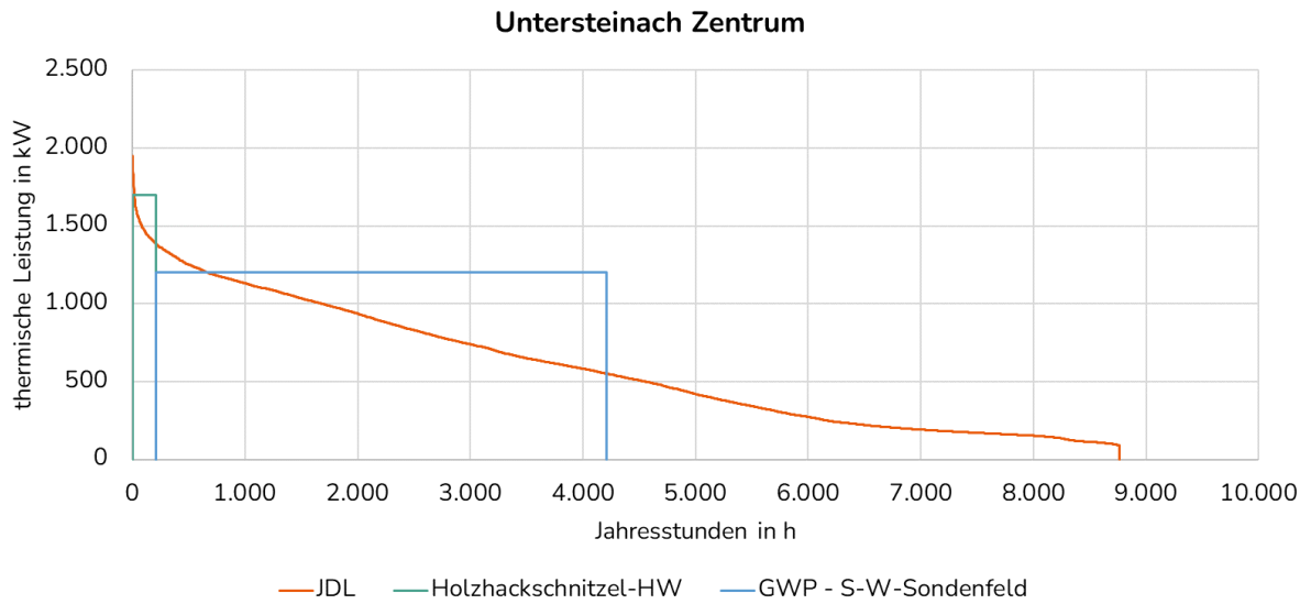
Abbildung 49: geordnete thermische JDL Untersteinach Zentrum mit Variante 2
