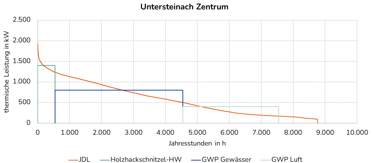
Abbildung 48: geordnete thermische JDL Untersteinach Zentrum mit Variante 1
