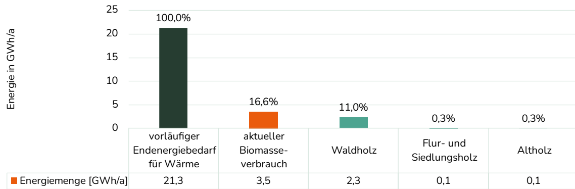
Abbildung 35: Endenergiepotenziale fester Biomasse
