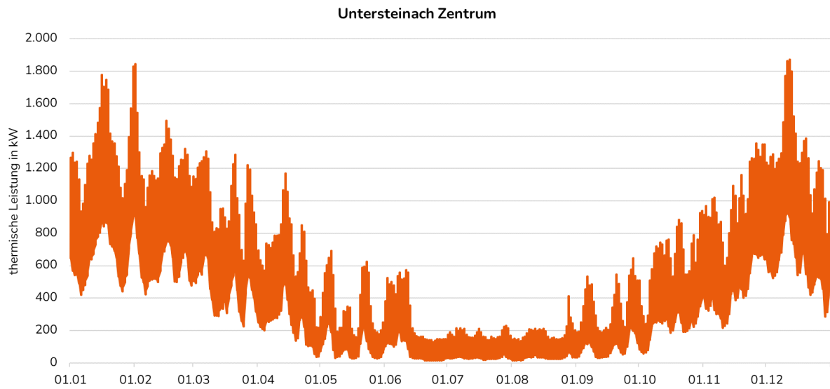
Abbildung 47: Lastprofil Wärmeverbrauch Untersteinach Zentrum inkl. Netzverluste
