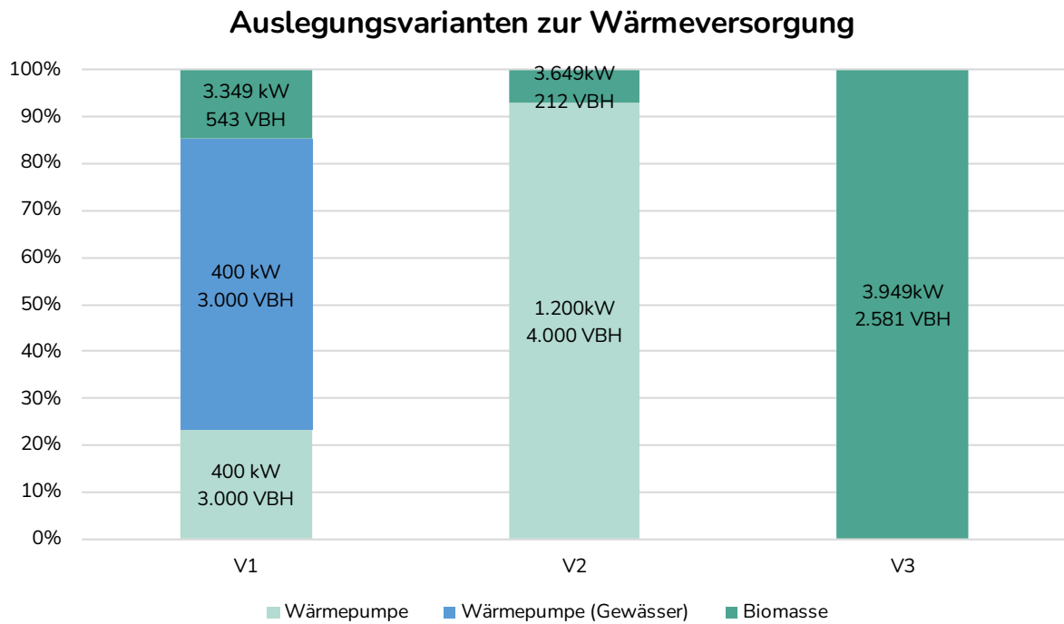
Abbildung 51: Vergleich Variantenauslegungen Untersteinach Zentrum
