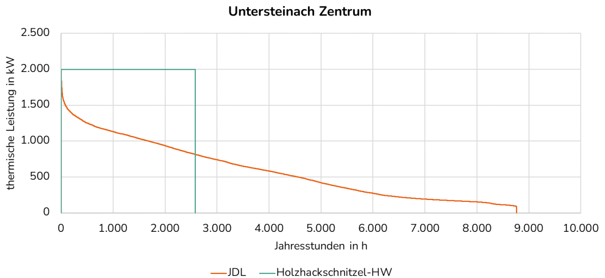
Abbildung 50: geordnete thermische JDL Untersteinach Zentrum mit Variante 3
